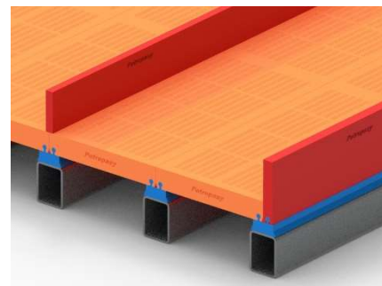
Sistema de fixação tipo Snapdeck
